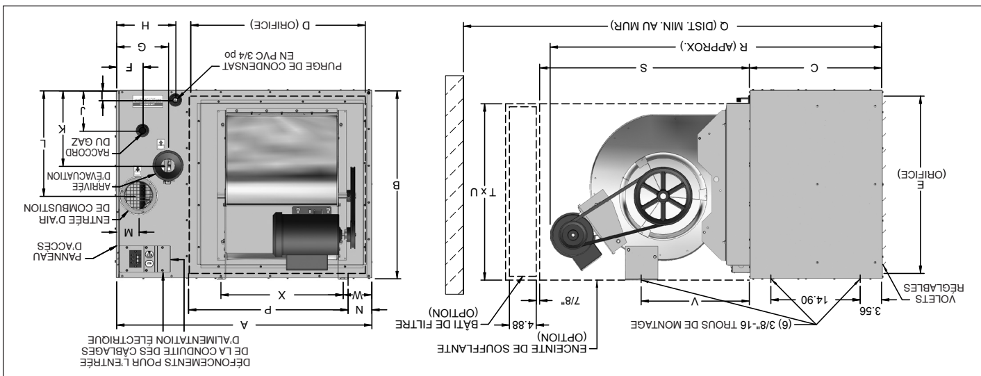
Figure 28.1 - Plans cotés - Modèle BTC
