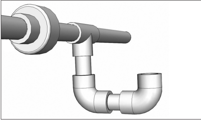
Figure 14.2 - Exemple de brise-vide
