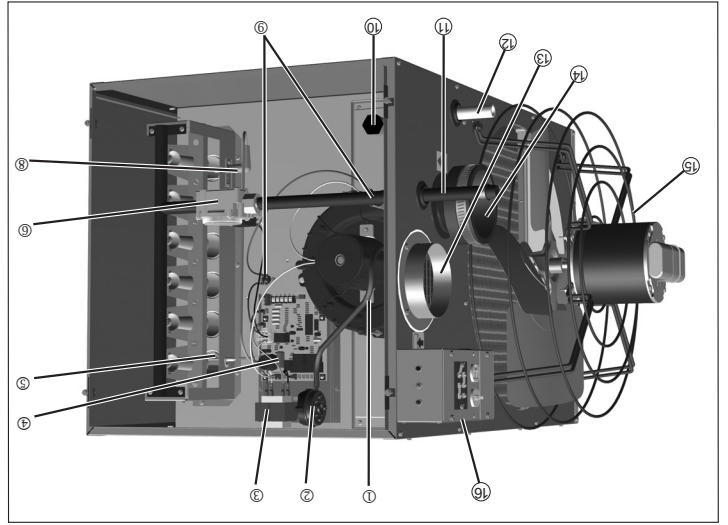
Figure 24.1 - Caractéristiques standard montées en usine
