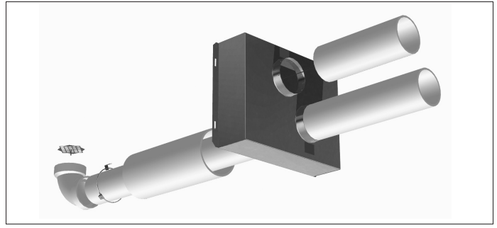
Figure 13.2 - Vue éclatée de la boîte adaptatrice
