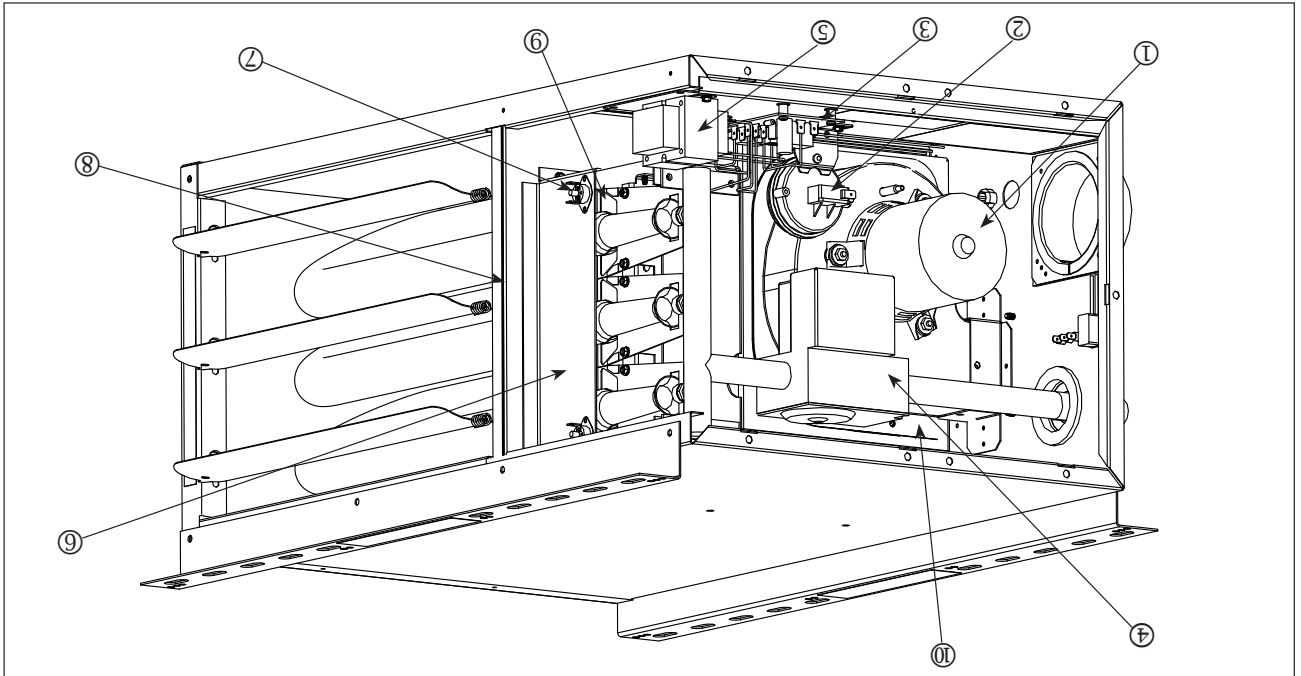
Figure 19.1 - Principaux composants des circuits de gaz, électriques, de sécurité et autres
