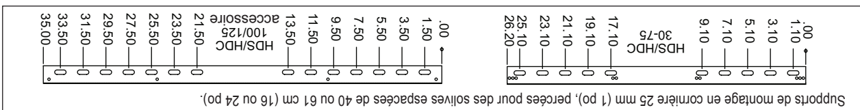
Figure 20.2 - Emplacements des fentes de cornière de fixation
