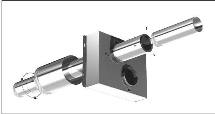
Figure 12.2 – Vue éclatée de la boîte adaptatrice
